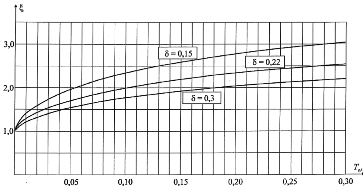
Рисунок 11.1* - Коэффициенты динамичности
