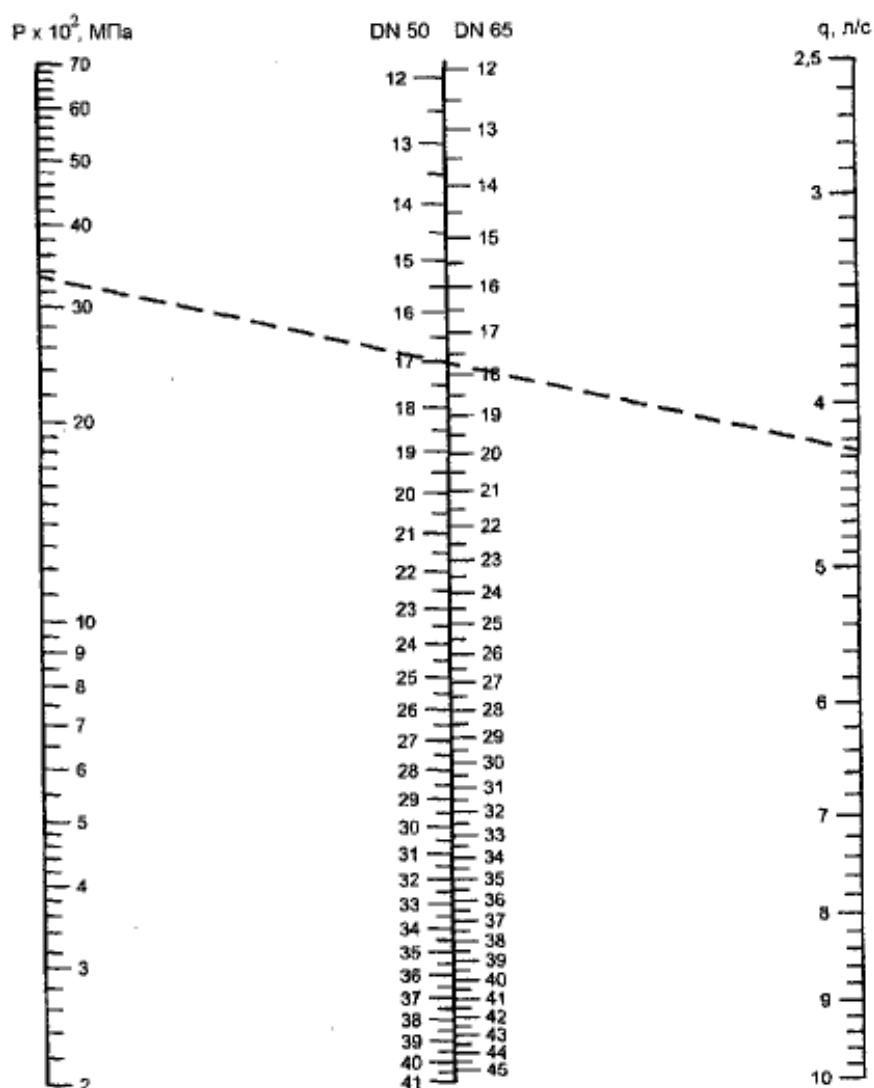
Номограмма для определения диаметра отверстия диафрагмы
