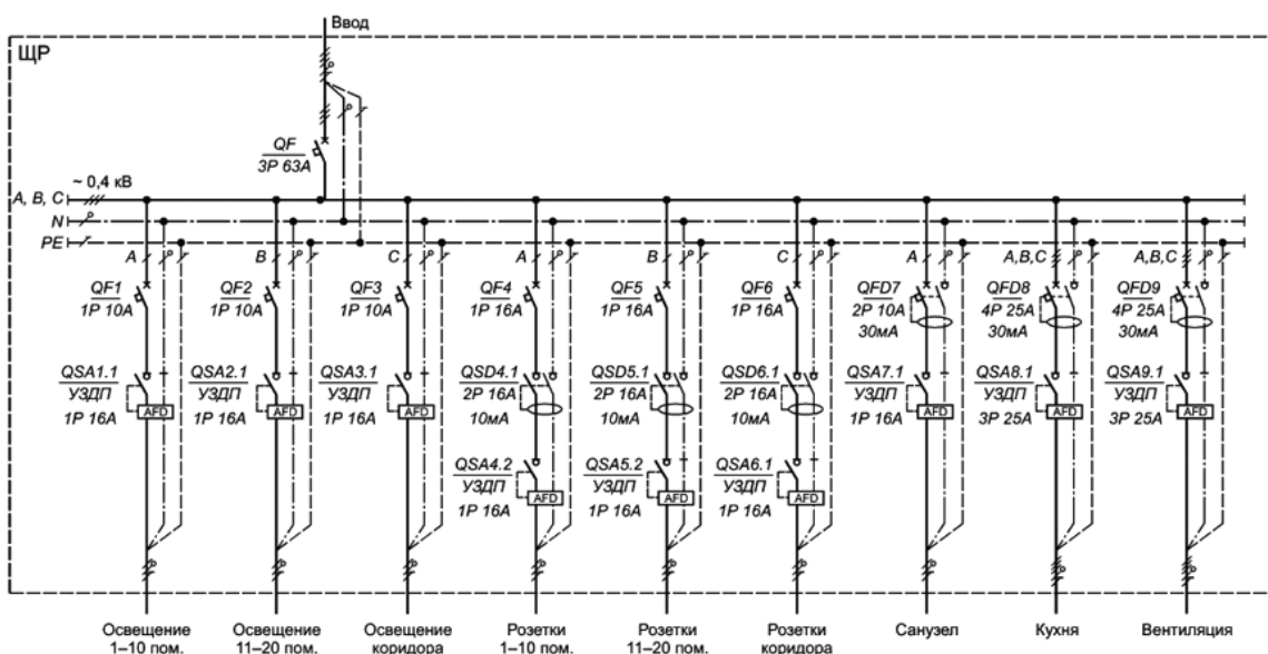
Рисунок В.9 - Применение УЗДП в электроустановке общественного здания. Трехфазная система
