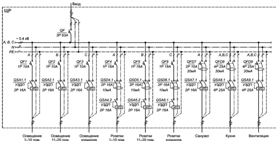
Рисунок В.10 - Применение УЗДП в электроустановке общественного здания. Трехфазная система электропитания с применением двухполюсных и четырехполюсных УЗДП
